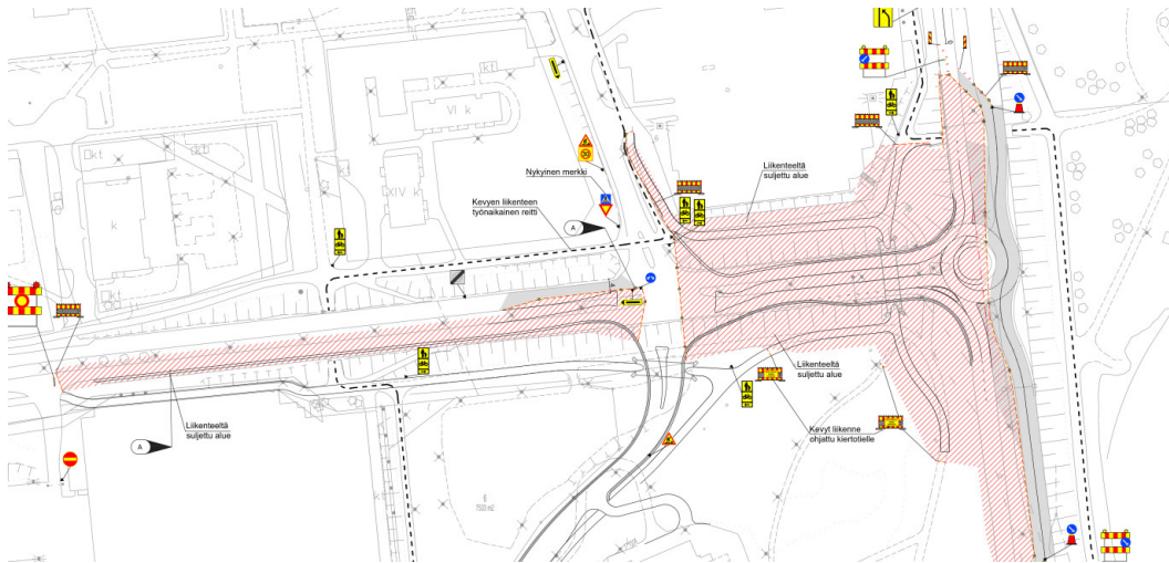
Liikenteenohjaussuunnitelma Keskuskadun ja Tainionkoskentie rakennusaikana
